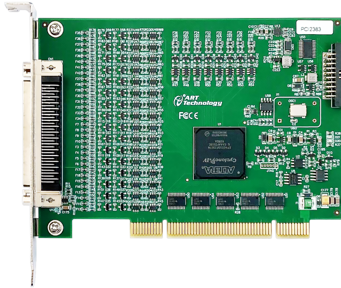
图 3-1-3 PCI2383 板卡正面图
