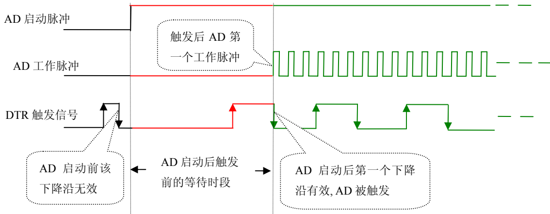
图 6.5 下降沿触发图例
