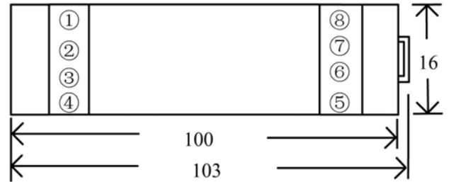
俯视图
