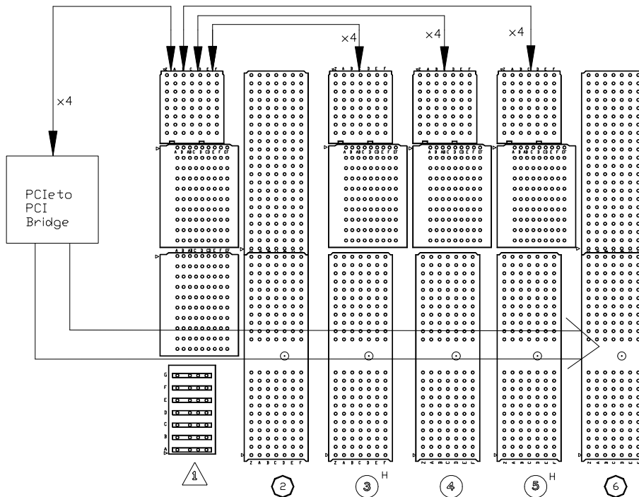
图 4 总线拓扑图
