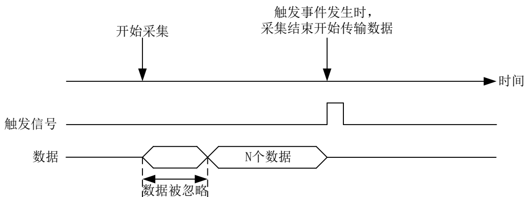
图 4-9-2-4 预触发
