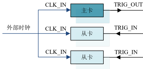
图 4-10-2 采用共同外时钟
