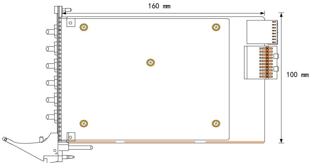
图 3-2-1 PXIe8922 板卡尺寸图
