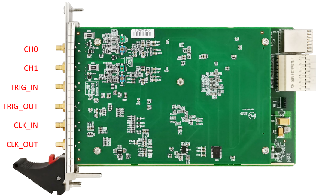
图 3-3-1 PXIe8922 产品外观图
