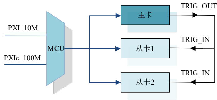
图 4-10-1 采用背板时钟信号作为时钟参考源
