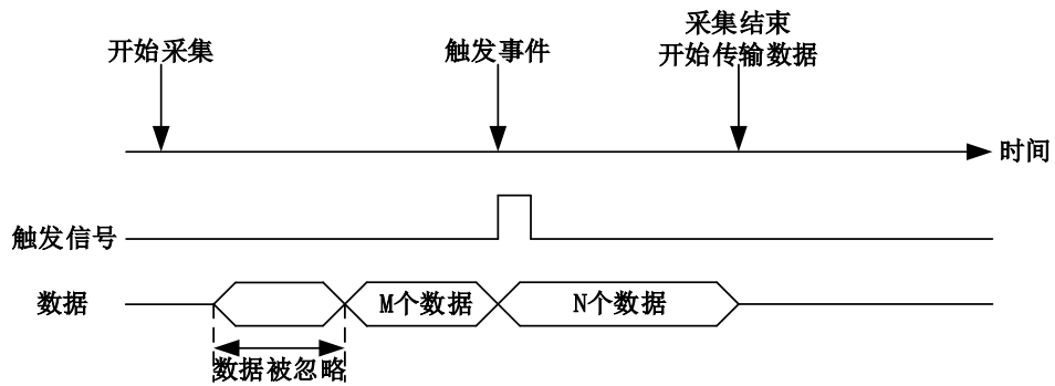
图 4-9-2-2 中间触发
