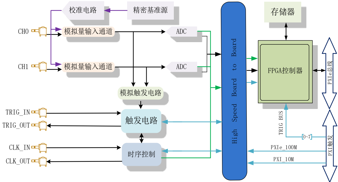
图 3-1-1 PXIe8922 系统框图
