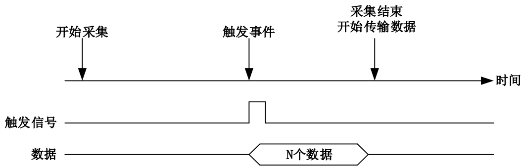
图 4-8-2-3 后触发
