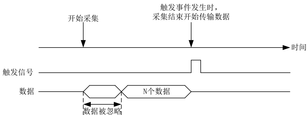
图 4-8-2-4 预触发
