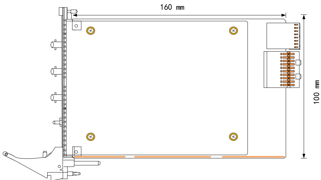
图 3-2-1 PXIe8910 板卡尺寸图
