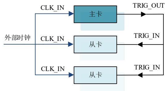
图4-9-2 共同的外时钟
