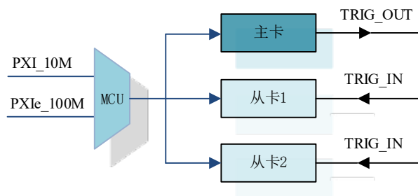
图 4-9-1 采用背板时钟信号作为时钟参考源
