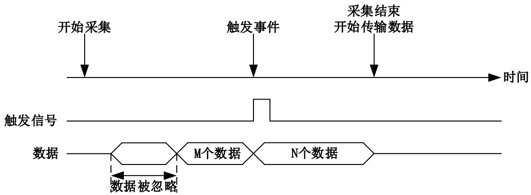
图 4-8-2-2 中间触发
