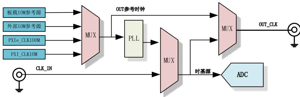
图 4-7-1 时基源框图
