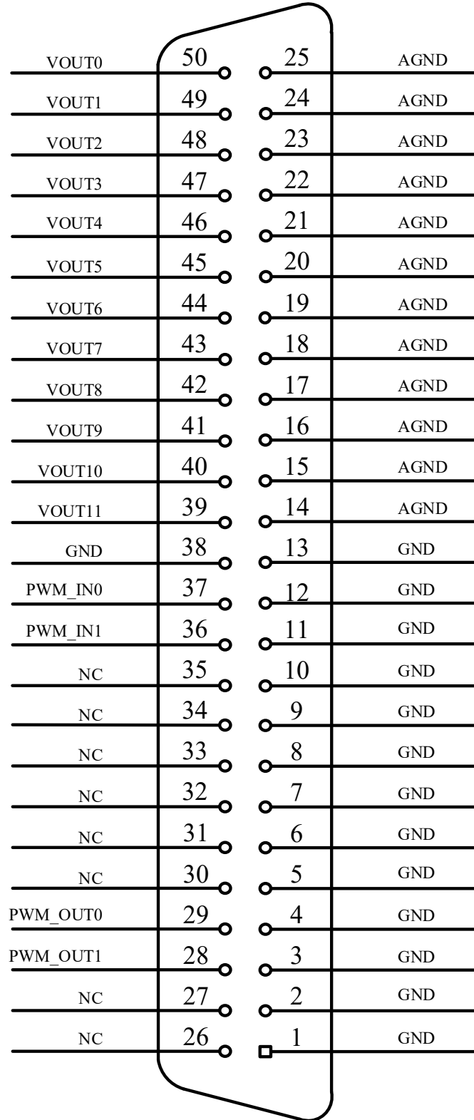
图 3-1-1 连接器定义图
