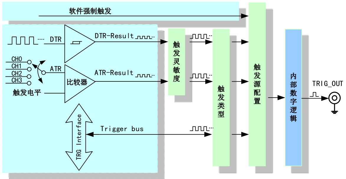
图 4-9-1 AI 触发功能框图
