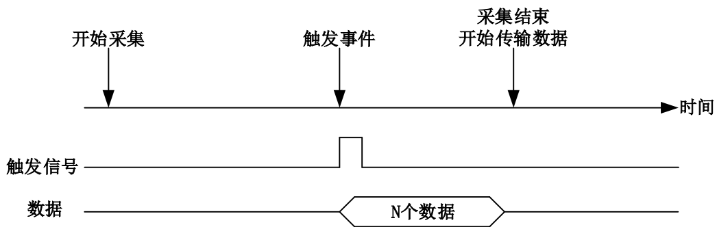
图 4-10-3 后触发
