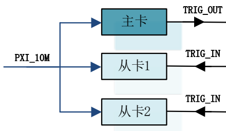
图 4-11-1 采用 PXI 机箱背板的 PXI_10M 时钟信号作为时钟参考源
