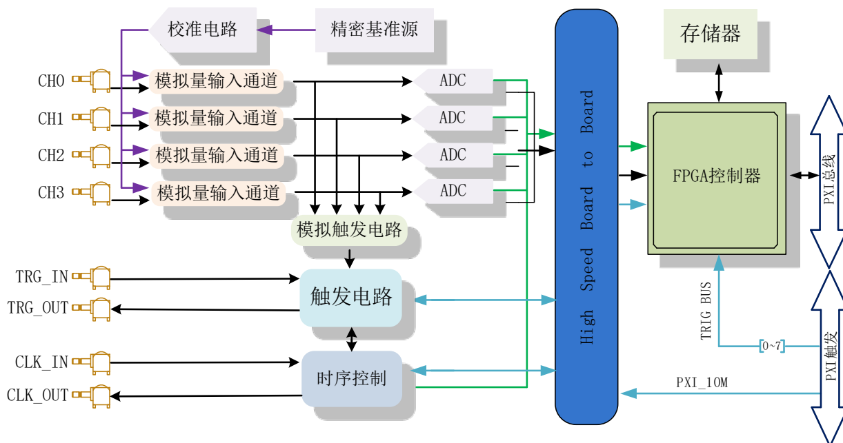
图 3-1-1 PXI8512B_14B_16B 系统框图
