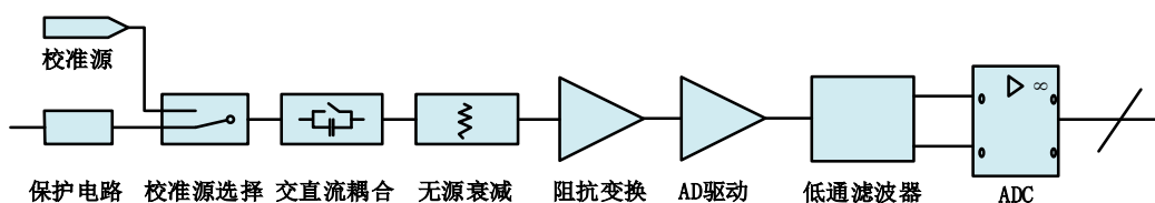
图 4-1-1 AI 功能框图
