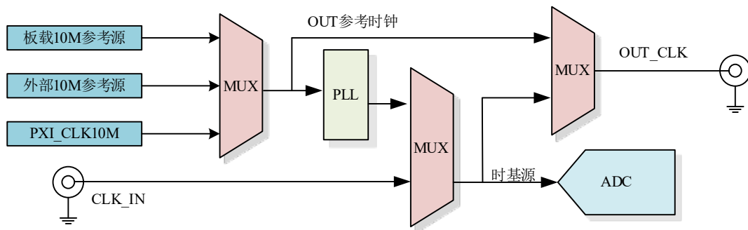
图 4-7-1 时基源框图
