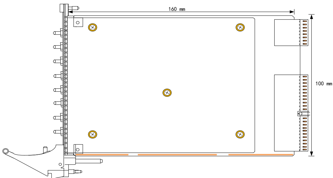
图 3-2-1 PXI8512B_14B_16B 板卡尺寸图
