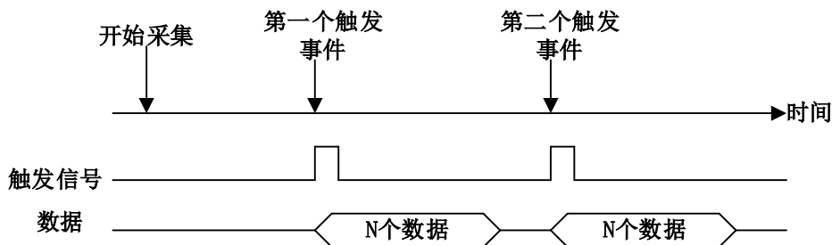
图 4-10-7 后触发和延时触发的重复触发
