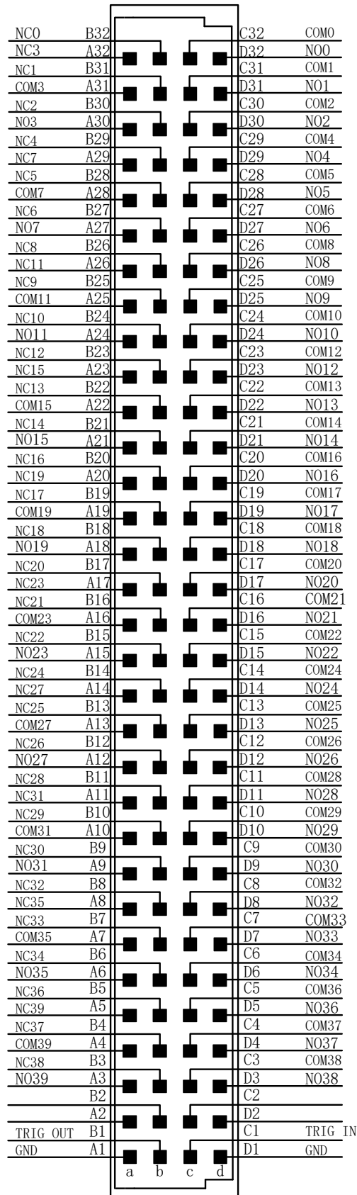
图 3-2-1 连接器引脚定义
