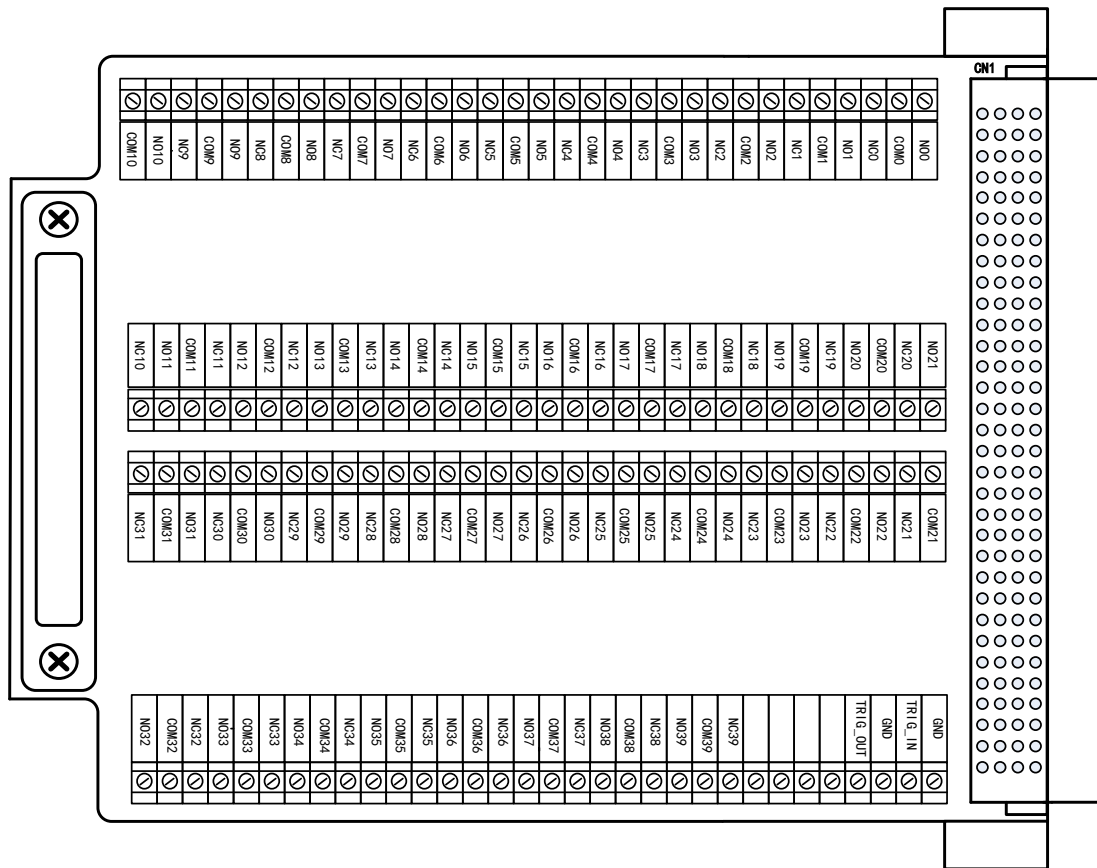
图 3-3-1 TB2604 端子盒接线定义图
