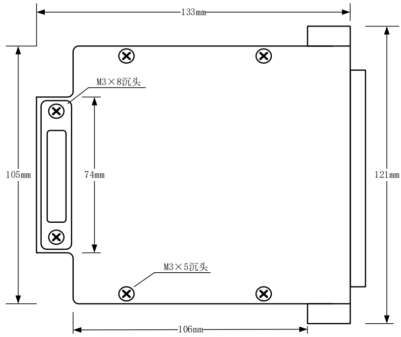
图 3-1-3 TB2604 尺寸图
