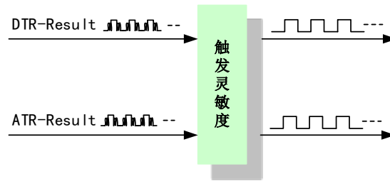
图 4-8-2 触发灵敏度
