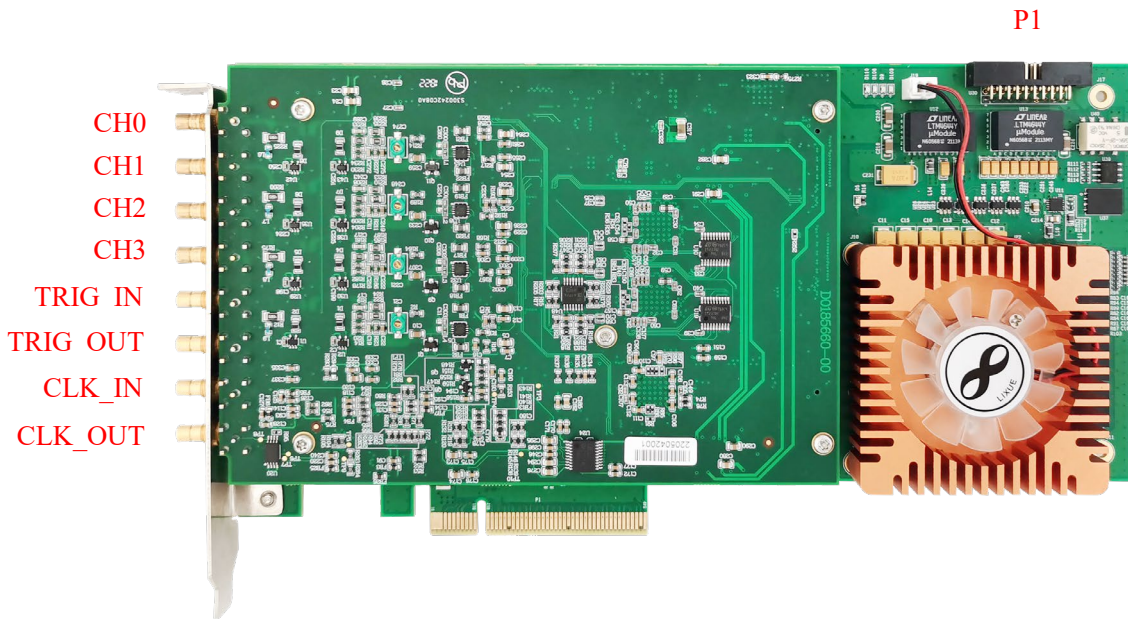
图 3-3-1 PCIe856x 产品外观图
