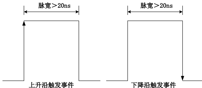
图 4-8-8 脉宽最小值图
