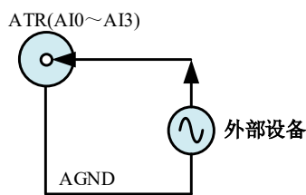
图 4-8-4 ATR 触发信号连接
