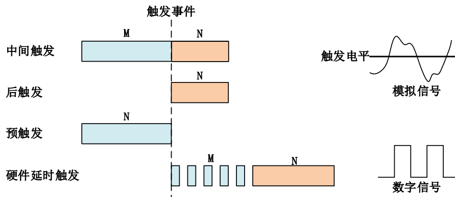
图 4-8-2-1 AI 触发模式
