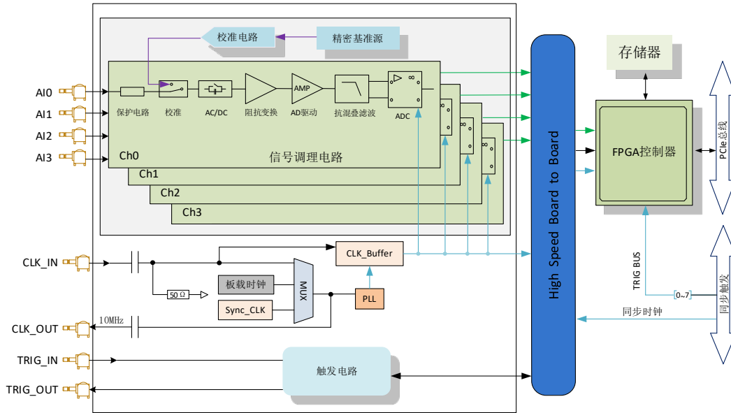
图 3-1-1 PCIe8911 系统框图
