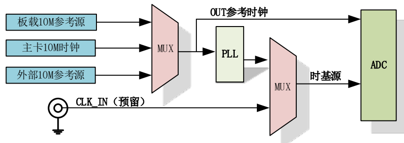
图 4-7-1 时基源框图
