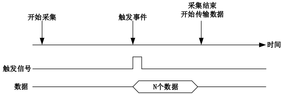
图 4-8-2-3 后触发
