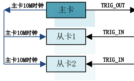
图 4-10-1 主从卡级联
