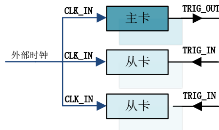
图 4-10-2 采用共同外时钟
