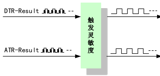
图 4-9-2 触发灵敏度
