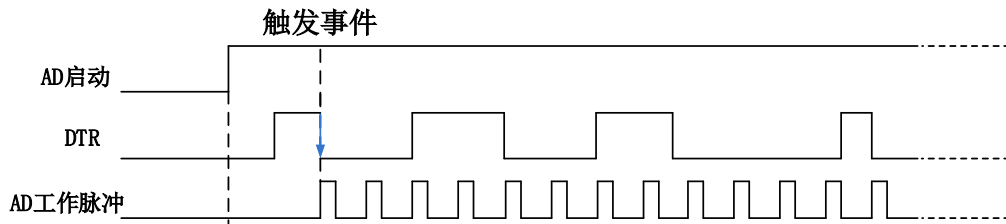
图 4-9-9 DTR 触发--下降沿触发
