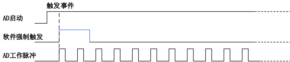
图 4-9-3 AI 软件触发
