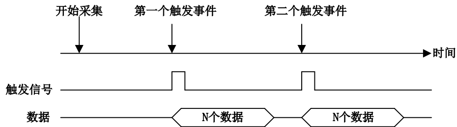
图 4-8-2-7 后触发和延时触发的重复触发
