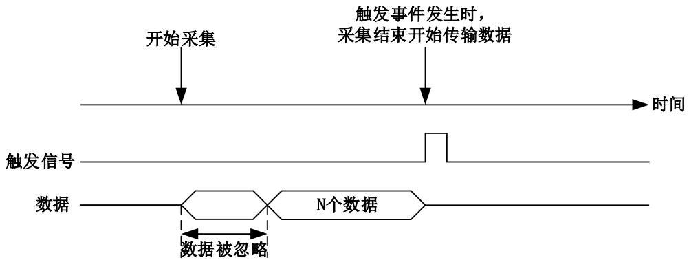
图 4-8-2-4 预触发
