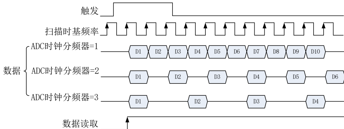
图 4-7-2 AI 抽样速率示意图
