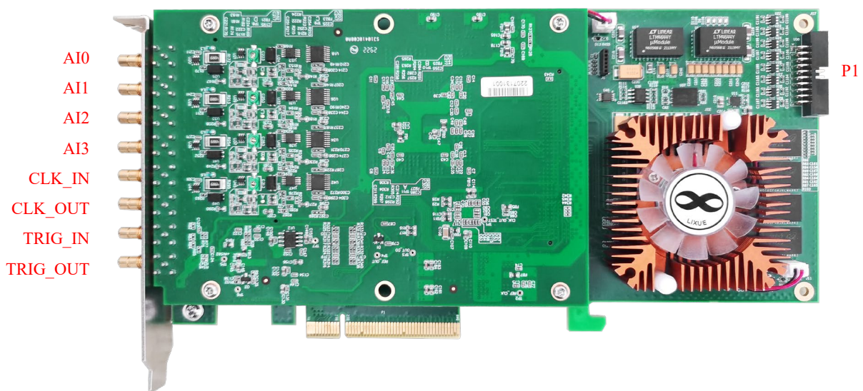
图 3-2-1 PCIe8911 产品外观图
