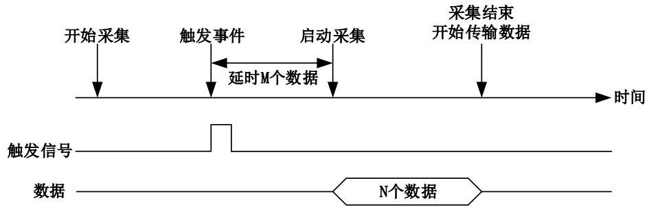
图 4-8-2-6 硬件延时触发
