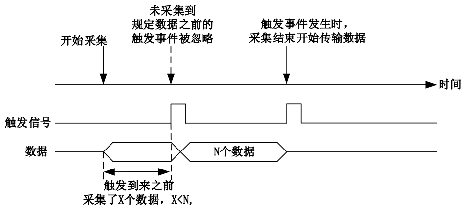
图 4-8-2-5 预触发--采集数据小于 N
