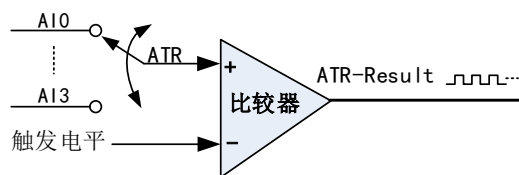
图 4-9-5 比较器
