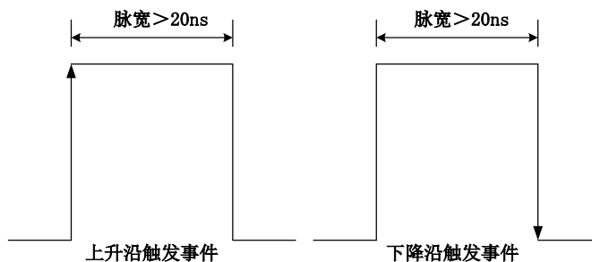
图 4-9-8 脉宽最小值图
