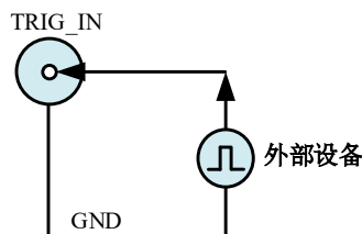
图 4-9-7 DTR 触发信号连接
