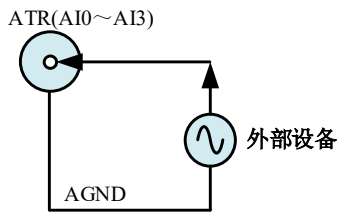
图 4-9-4 ATR 触发信号连接
