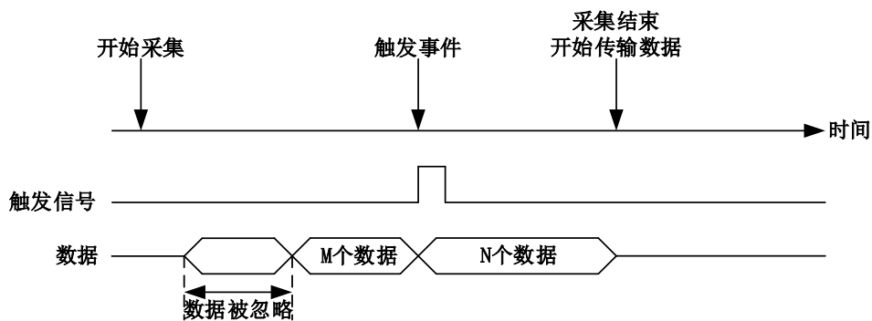
图 4-8-2-2 中间触发
