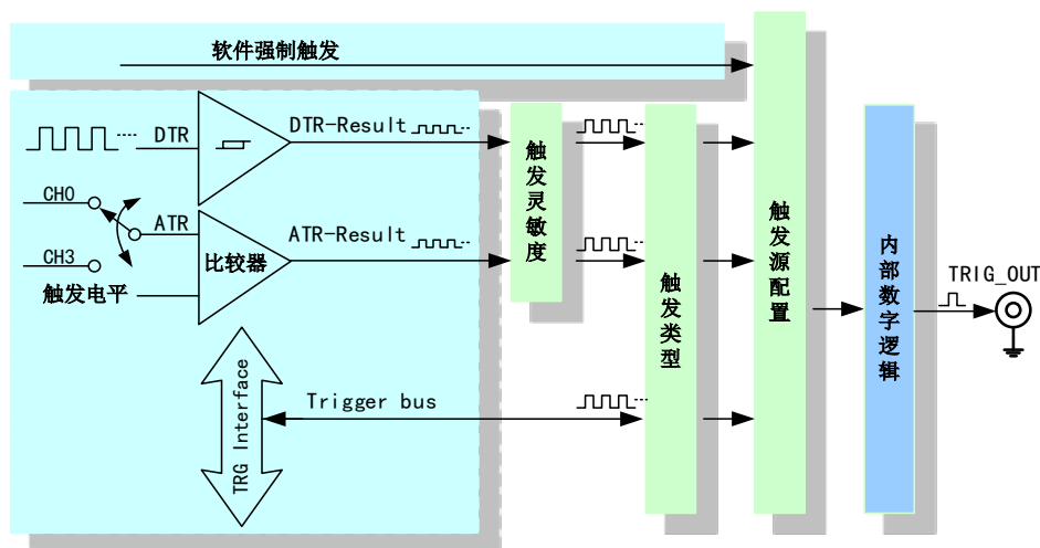
图 4-9-1 AI 触发功能框图
