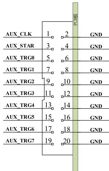
图 3-3-1 P1 管脚定义
