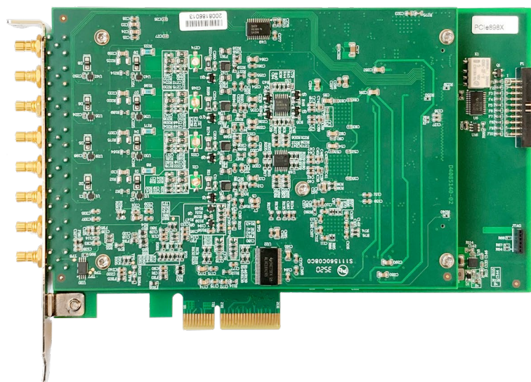
图 3-3-1 PCIe85X6 产品外观图
