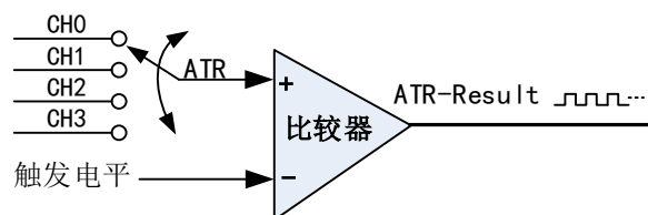
图 4-8-5 比较器
