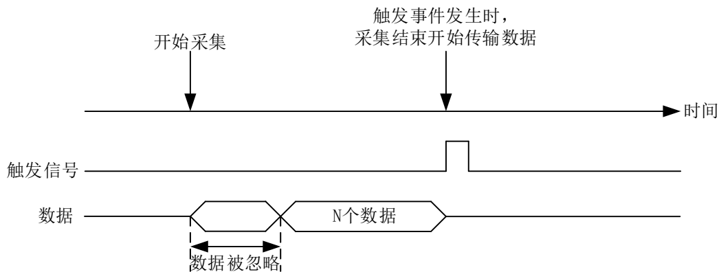
图 4-9-2-4 预触发
