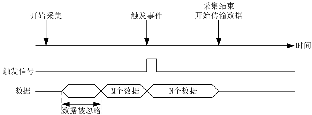
图 4-9-2-2 中间触发
