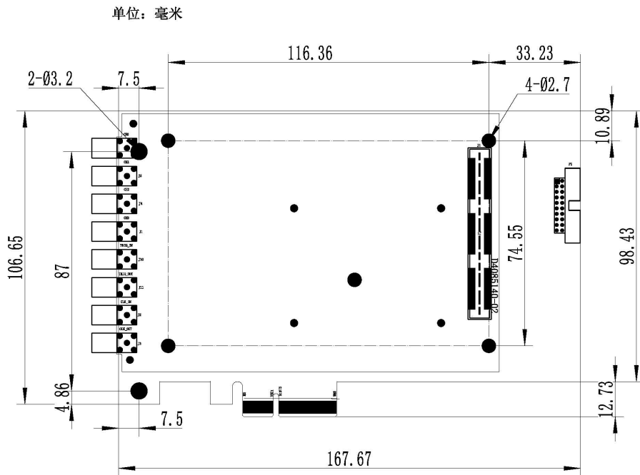
图 3-2-1 PCIe85X6 板卡尺寸图
