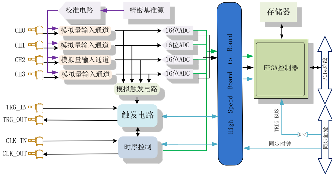
图 3-1-1 PCIe85X6 系统框图
