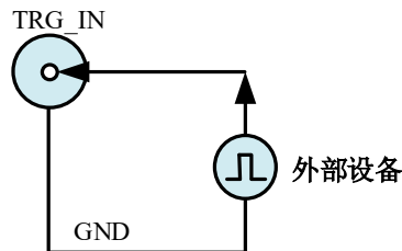
图 4-8-7 DTR 触发信号连接
