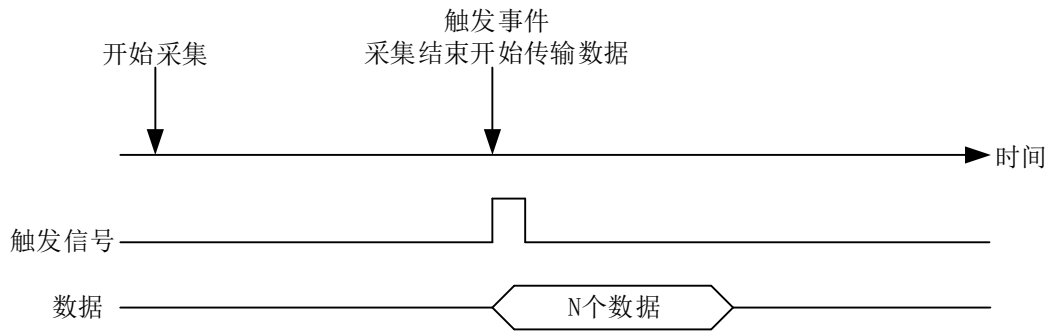
图 4-9-2-3 后触发
