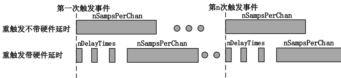
图 4-7-5 AI 重触发
