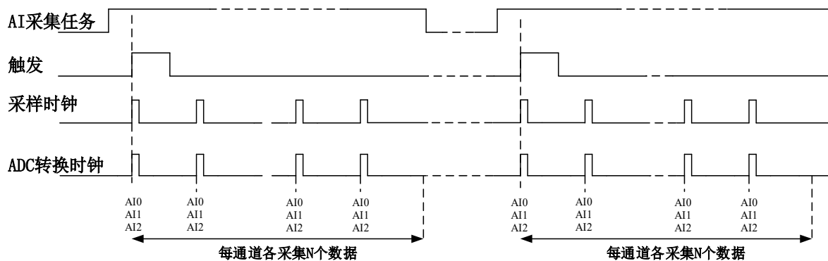
图4-6-2 有限点采样
