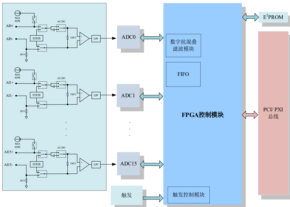
图 2-2-1 8816 系统框图示意
