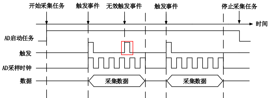
图 4-7-6 重触发
