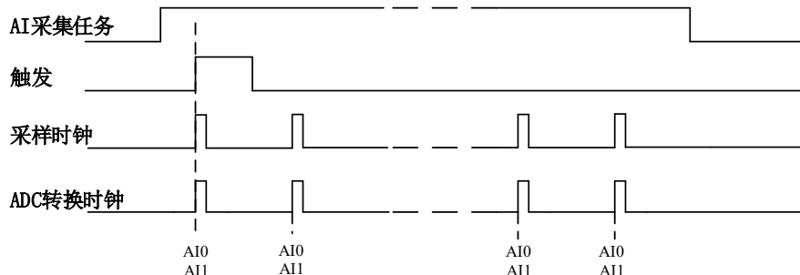
图4-6-3 连续采样
