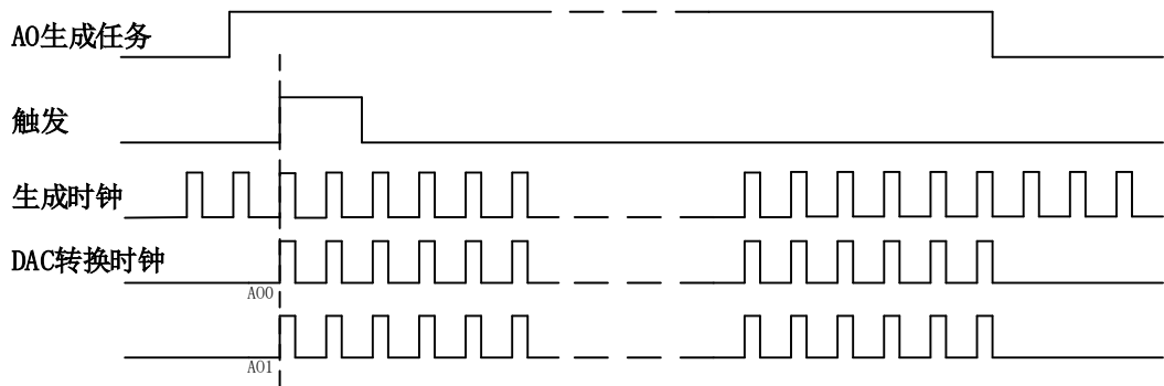
图5-5-3 内、外时钟连续采样
