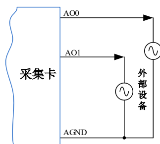
图5-2-1 AO模拟量输出连接
