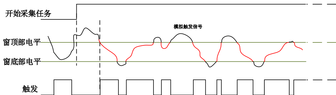
图6-2-8 模拟窗触发--入窗
