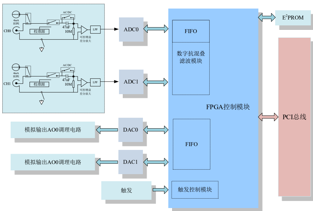
图 2-1-1 PCI8822 系统框图
