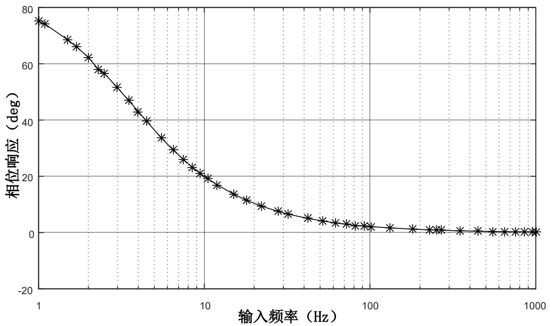
图 2-2-2 交流耦合电路的相位响应(1Hz~1kHz)
