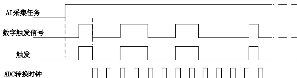
图 6-1-2 开始触发分类
