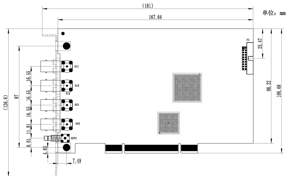
图 3-2-1 PCI8822 板卡尺寸图
