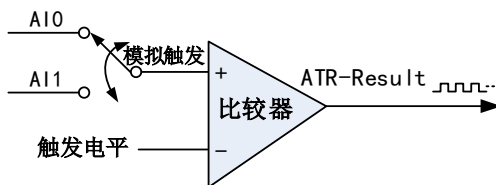
图6-2-5 比较器
