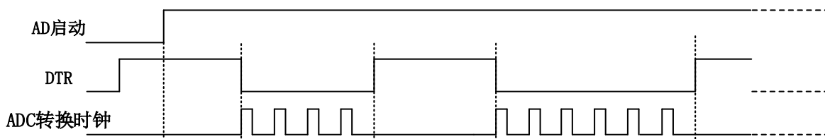
图 6-1-6 暂停触发—高电平暂停
