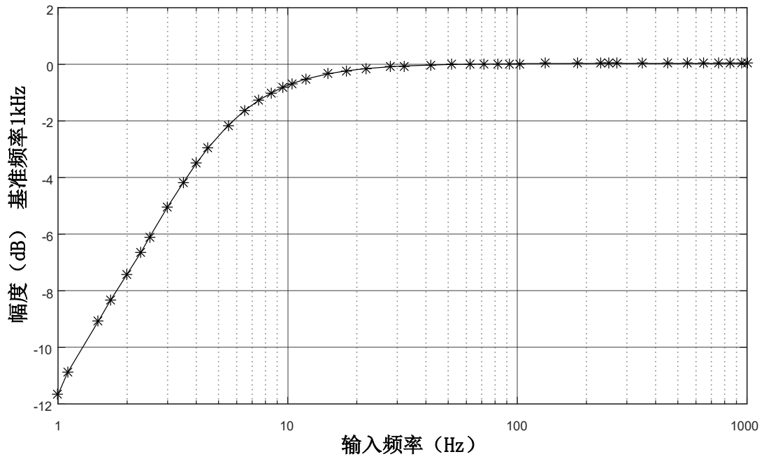
图 2-2-1 交流耦合电路的幅度响应(1Hz~1kHz)
