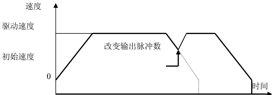
图 2.1.2 在匀速段增加脉冲数
