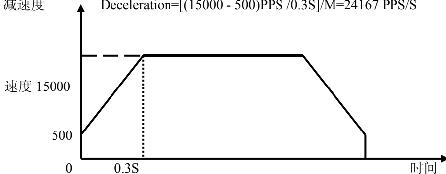
图 2.2.3 定长脉冲驱动模式
