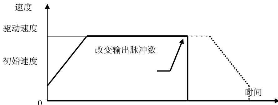
图 2.1.4 减少脉冲数
