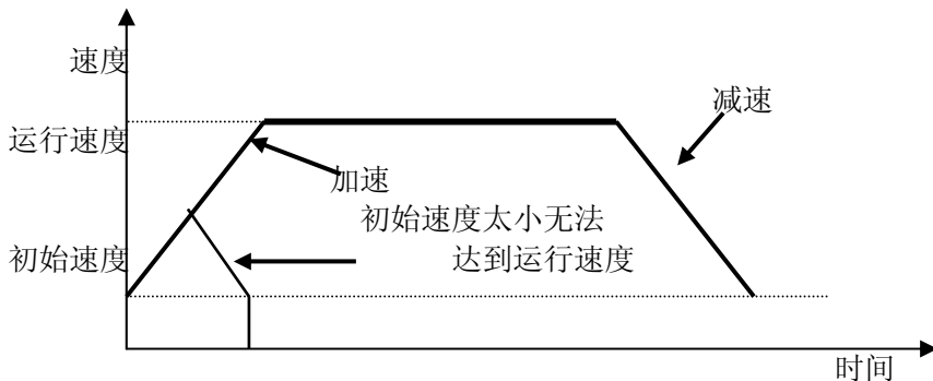
图 2.2.2 直线加/减速
