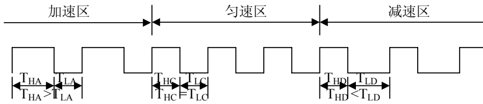
图 2.2.5 加/减速过程中脉冲宽度的比较
