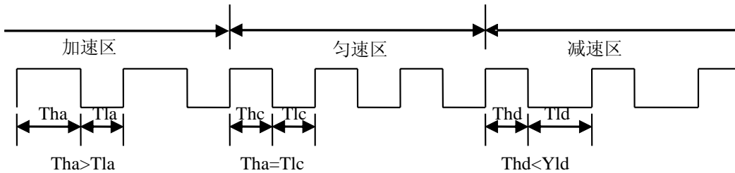
图 2.2.5 加/减速过程中脉冲宽度的比较
