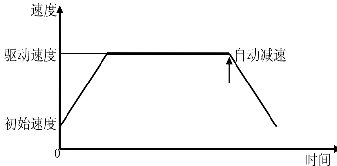
图 2.1.1 定长脉冲驱动模式
