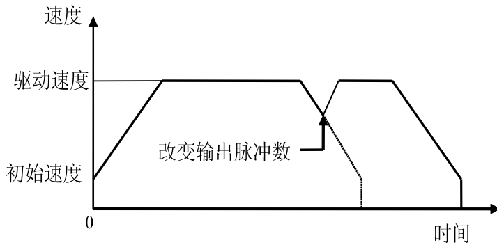
图 2.1.3 在减速段增加脉冲数
