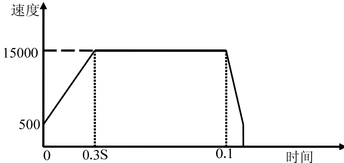
图 2.2.4 定长脉冲驱动模式加/减速度不同
