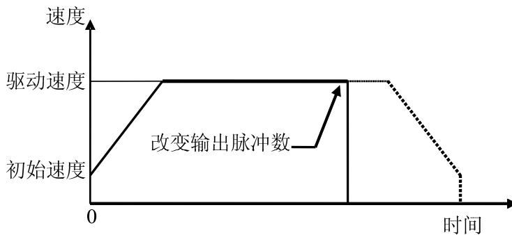
图 2.1.4 减少脉冲数
