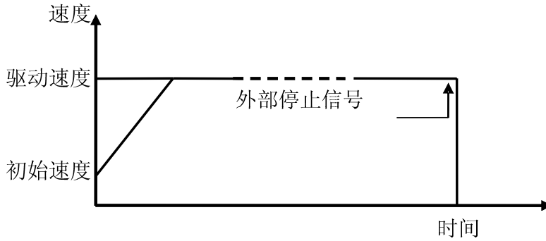
图 2.1.6 连续脉冲驱动
