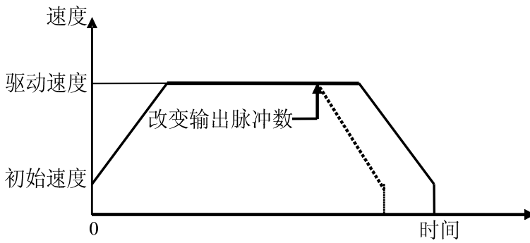
图 2.1.2 在匀速段增加脉冲
