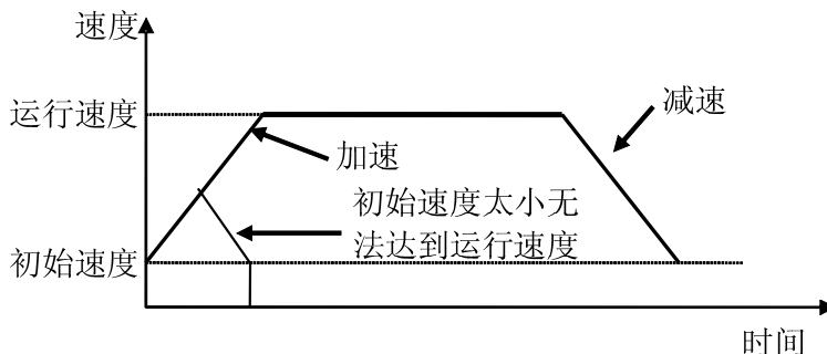
图 2.2.2 直线加/减速
