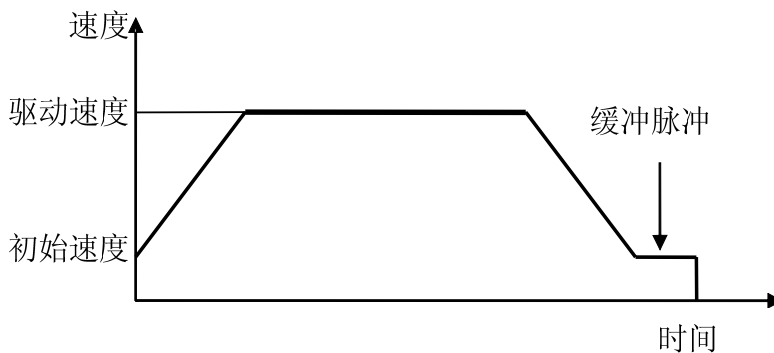
图 2.1.5 定长方式下的缓冲脉冲
